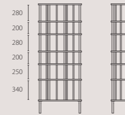
LE756 H 1900 W 750 D 320
