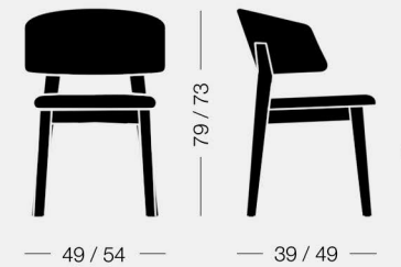
Wrap 6C60 7,2 kg 0,23 m³ 1 pz
