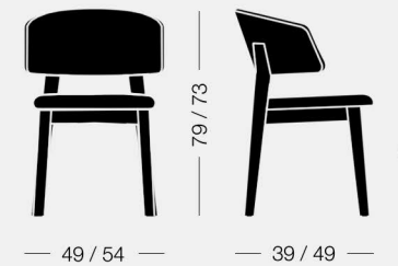
Wrap Wood 6C61 7,2 kg 0,23 m³ 1 pz
