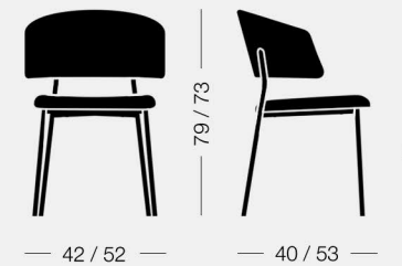
Wrap Steel 6C70 5,4 kg 0,24 m³ 1 pz
