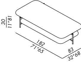
tavolo basso / low table 85180
