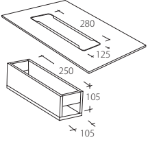
TKB4 Kabelgenomföring med elbrunn. Lösa lock. Cable slot with box. For socket and leads. Loose covers. Bord Table Tailor, Thinner, Trippo. Endast rektangulära skivor till Bouquet, Cross, Locus och Ypsilon. Only for rectangular tops to Bouquet, Cross, Locus and Ypsilon.
