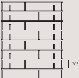
KOMB 10 7 x SIA 205135, 1 x SIB 205 H 1896 W 1544 D 330
