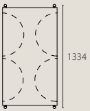
KC1 12570 H 725 L 1250 W 700
